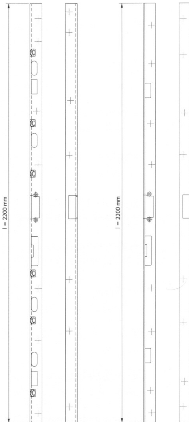
Abb. Schließbleiste für KfV AS 2606
