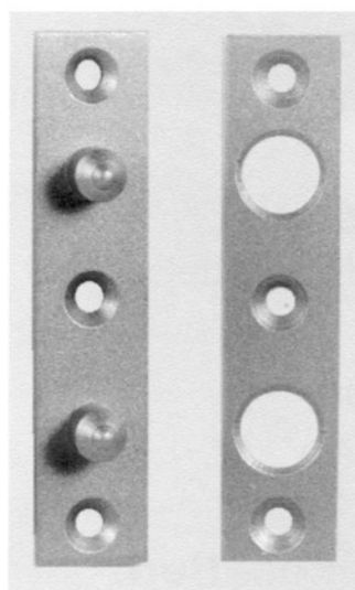
Bandsicherung TYP 3 Ausführung FS Ankerblech und Gegenblech wie Ausführung FS MA jedoch nicht für Maueranker vorgerichtet
