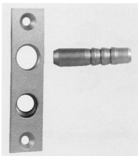
Bandsicherung TYP 1 , Ausführung FS MA Ankerblech 22 x 3 x 90 mm, vorgerichtet für Maueranker Zapfen zum Einbohren, Ø 11 x 50 mm
