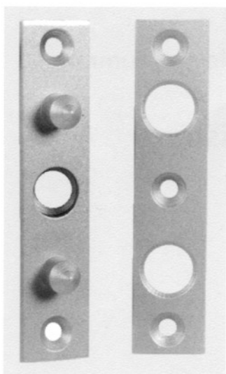
Bandsicherung TYP 3 Ausführung FS MA Ankerblech 22 x 3 x mm mit 2 eingienieteten Zapfen, vorgerichtet für Maueranker Gegenblech mit 2 Zapfenbohrungen
