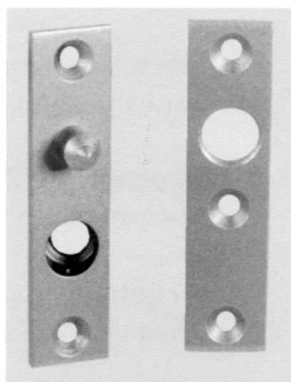
Bandsicherung TYP 2 , Ausführung FS MA Ankerblech 22 x 3 x 90 mm, vorgerichtet für Maueranker mit eingienieteten Zapfen, Gegenblech mit Zapfenbohrung
