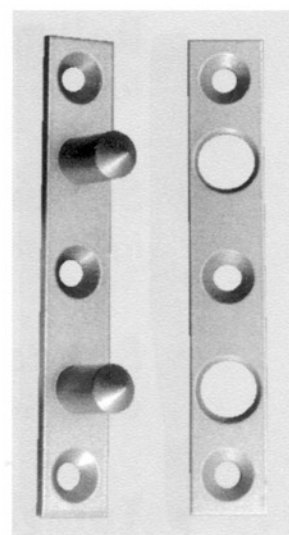
Bandsicherung TYP 3 Ausführung für Euronut Ankerblech 16 x 3 x 100 mm mit 2 verlängerten Zapfen Gegenblech mit 2 Zapfenbohrungen
